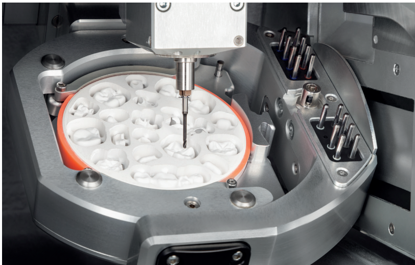
5-achsige Bearbeitung mit 16-fach Werkzeugwechsler
